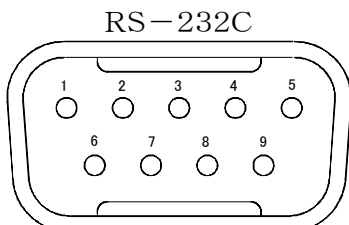
D-Sub 9ピン オス (コネクタ側面から見た図)
